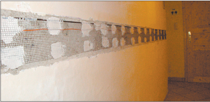
Anbringen des Netzgitters (Pluspol) zur Trockenlegung der Mauer.
